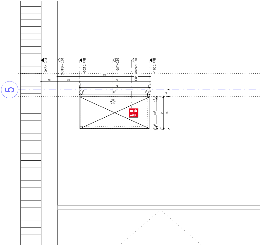
Vertikalschnitt S1-S1; M1:20
