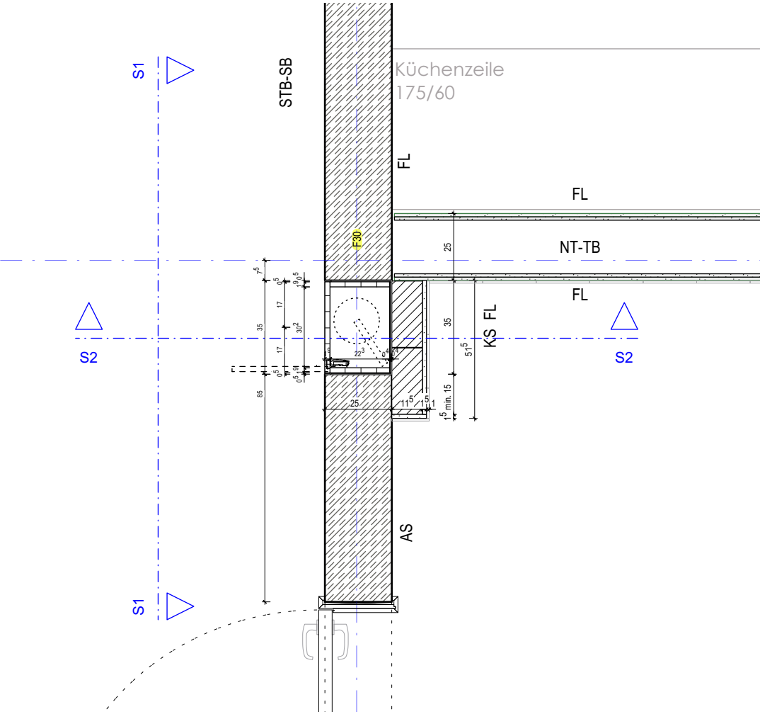
Horizontalschnitt; M1:20
