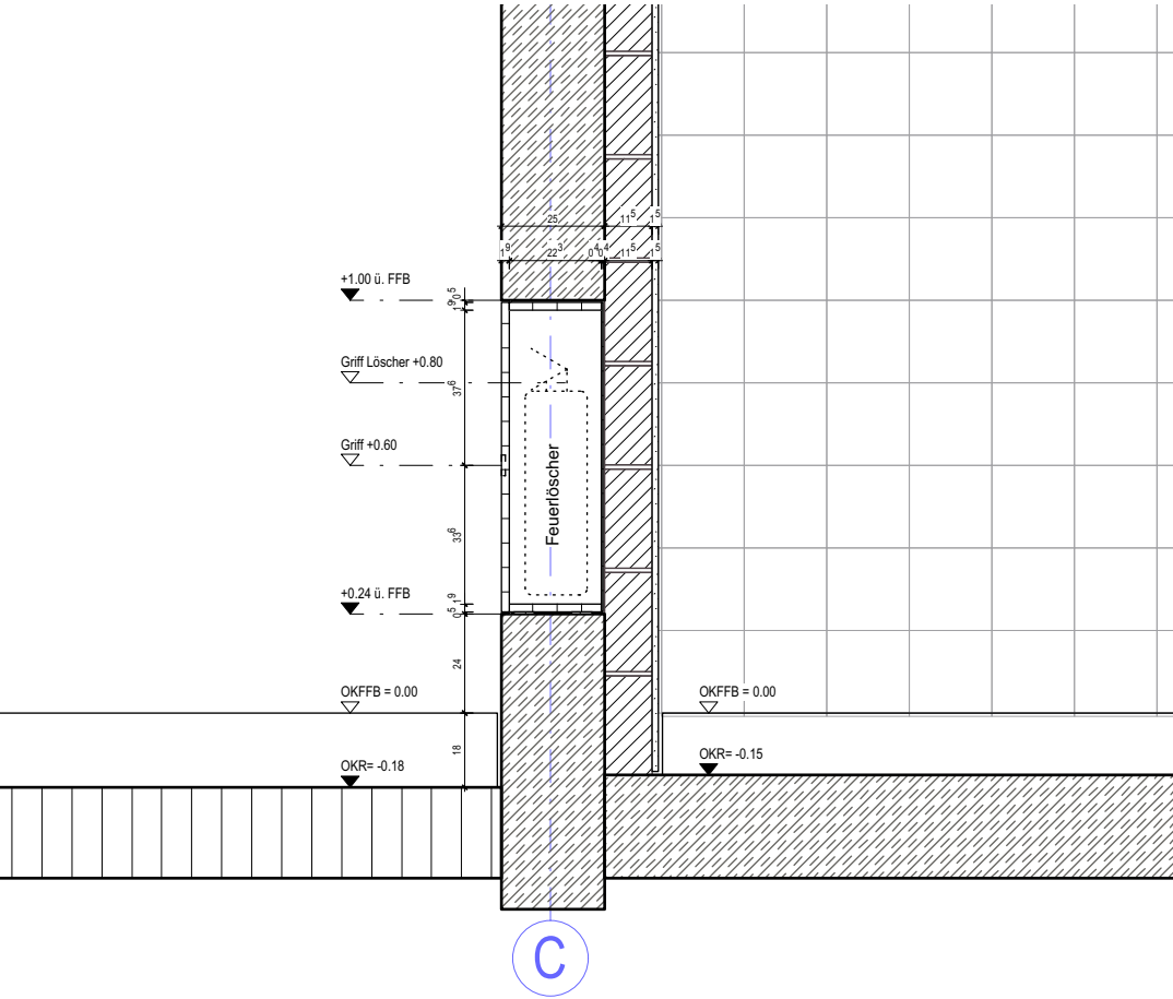
Vertikalschnitt S2-S2; M1:20
